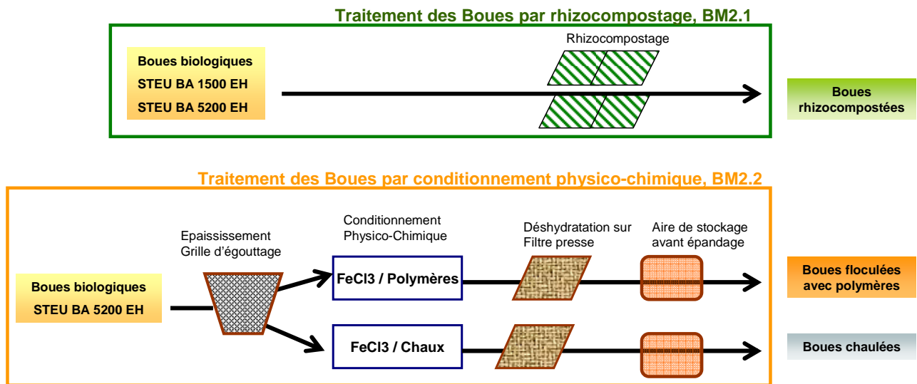
Figure 4. Découpage schématique des filières de traitement des boues
