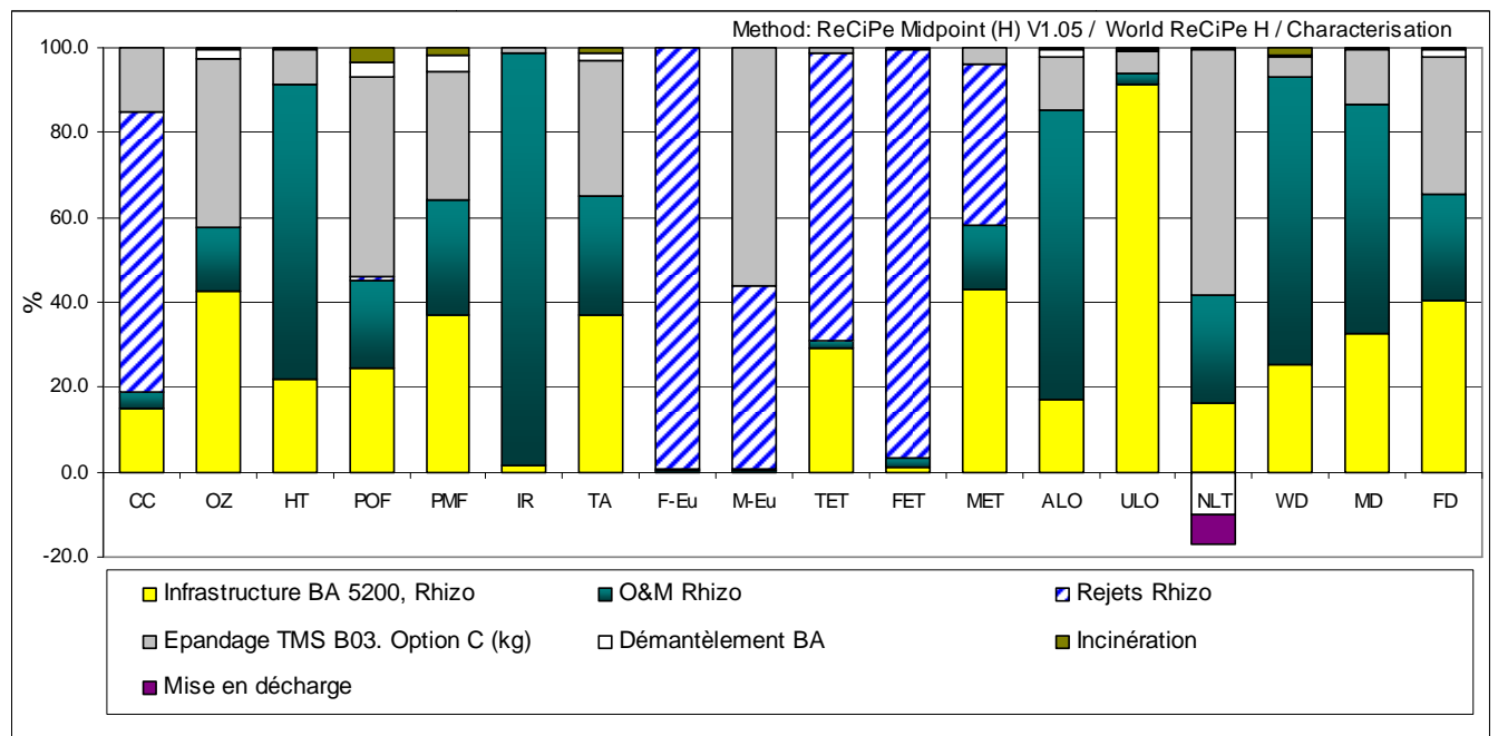
Figure 10. Diagramme de contribution, système BA Rhizo 5200 EH
