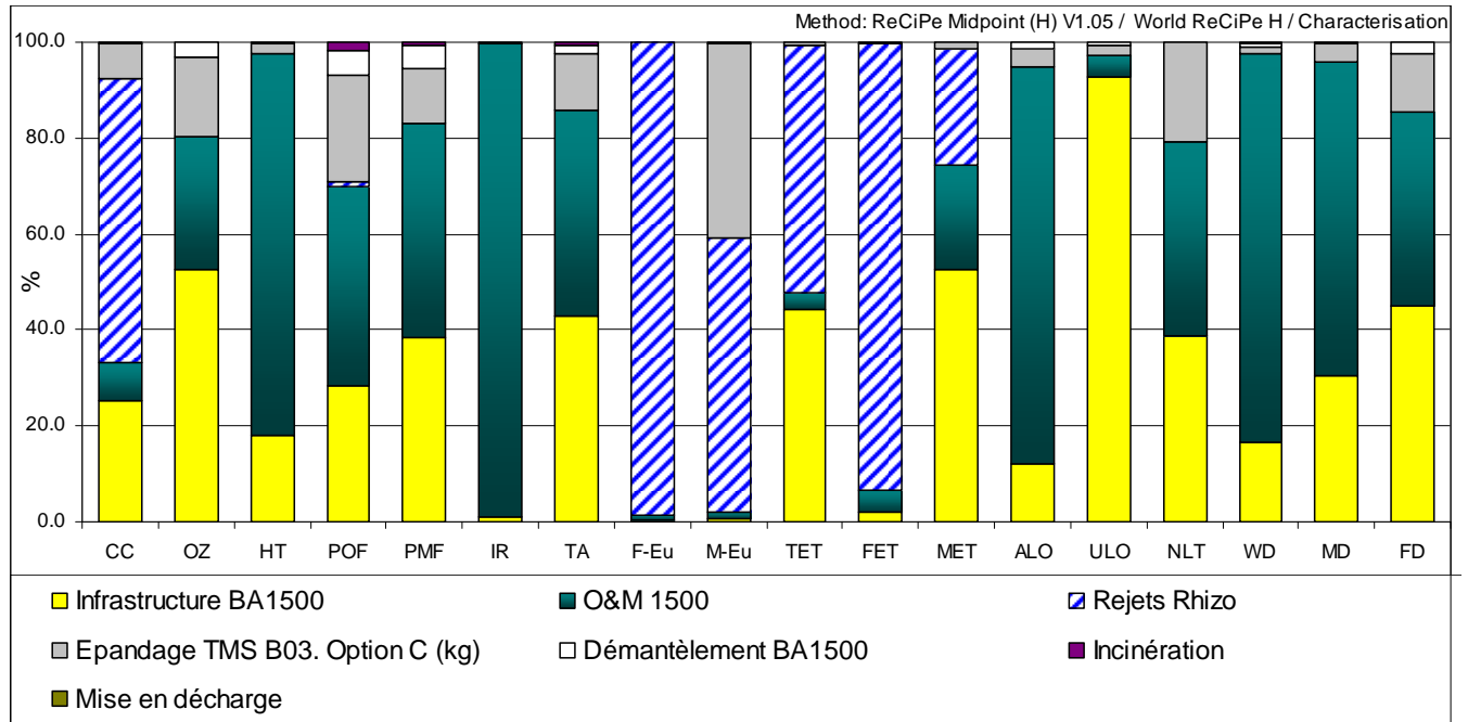
Figure 9. Diagramme de contribution, système BA Rhizo 1500 EH
