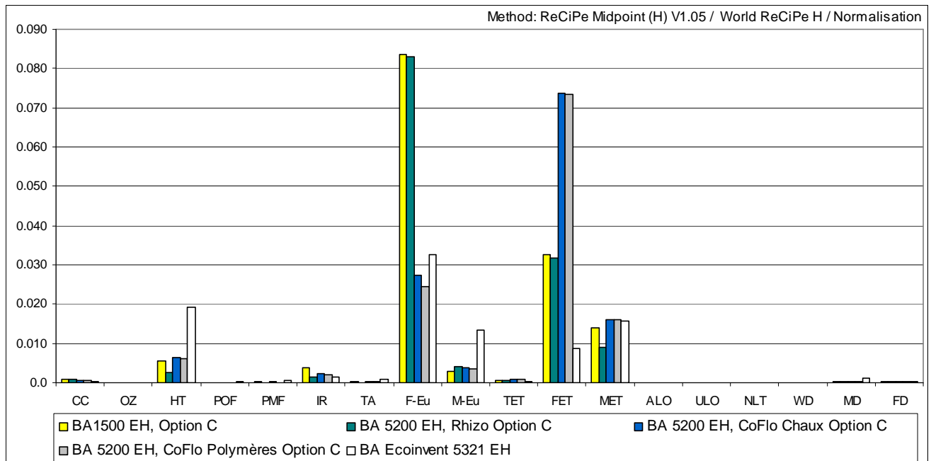
Figure 14. Contributions normalisées des systèmes BA modélisés
